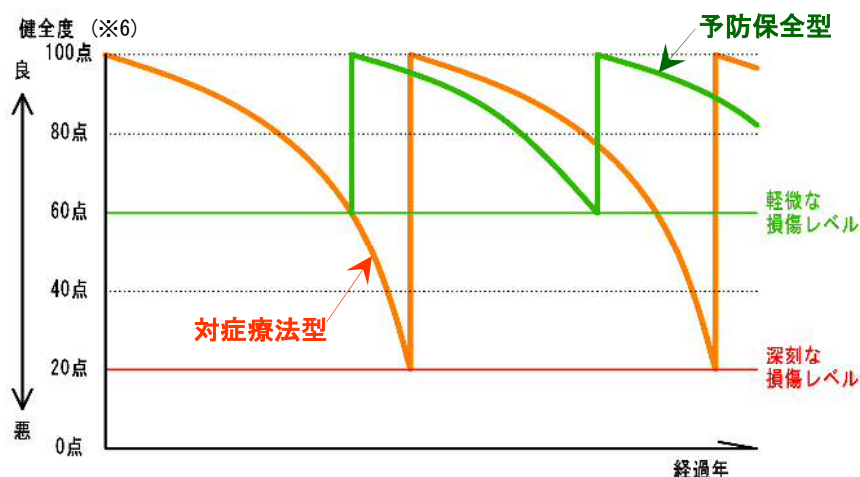
予防保全型と対症療法型の修繕サイクルイメージ
